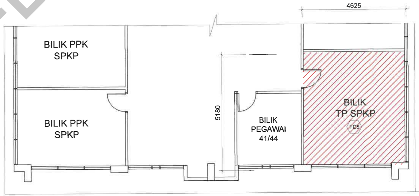
PELAN LANTAI (LOKASI 'B') SKALA : 1 : 100
